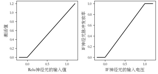
(a) ReLU 的激活值变化 (b) IF 神经元脉冲发放率变化
