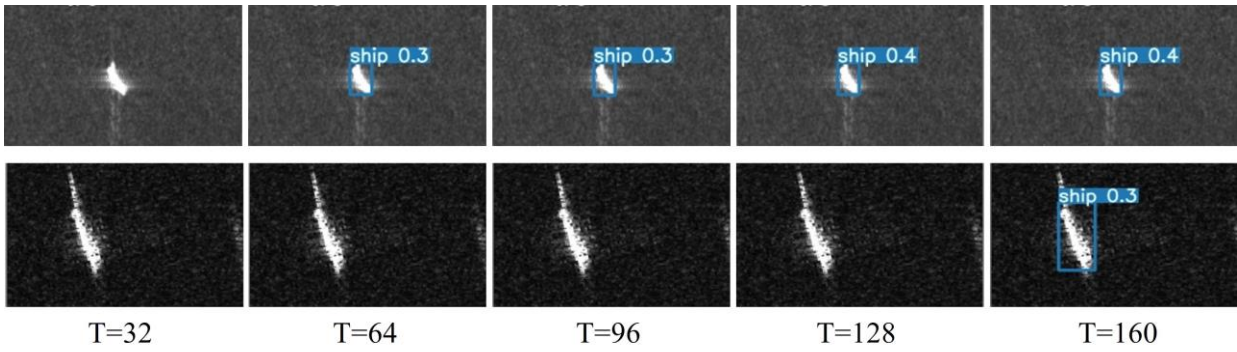
图 6 不同时间步下转换的类脑脉冲神经网络检测效果
