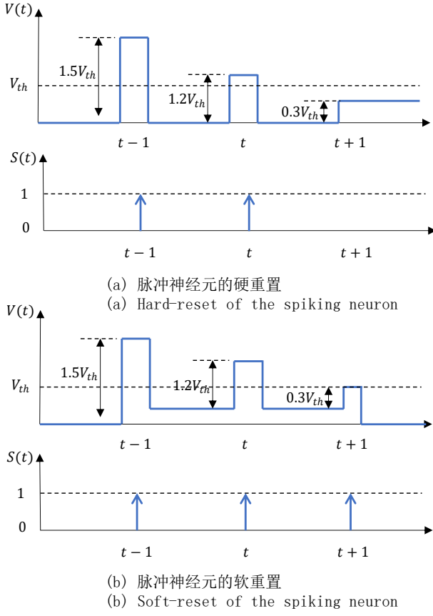
图2 在脉冲神经元的两种重置方式下，膜电位变化与神经元放电的示意图
