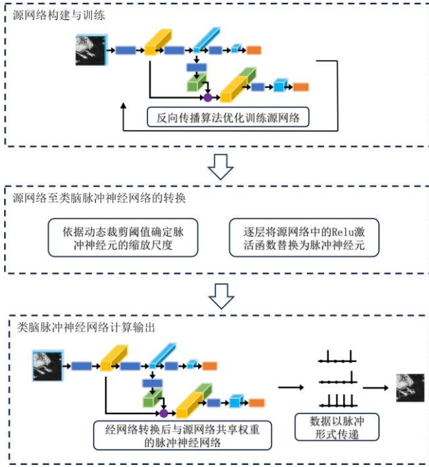
图 1 算法流程图
