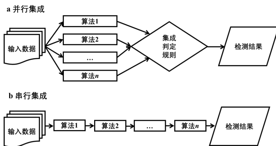
图1 多变化检测算法集成(修改自 Bullock 等, 2020a)
