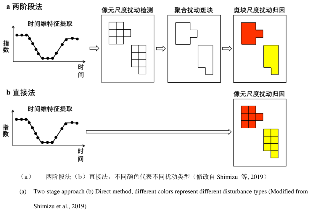
图2 森林多类型扰动归因方法
