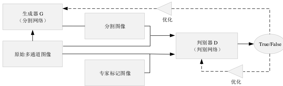
图 3. 海雾检测模型架构
