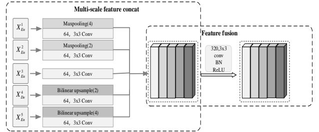
图 7. 解码器第三层多尺度特征拼接与特征融合结构
