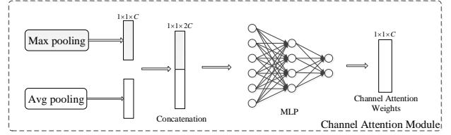
图 6. 通道注意力模块
