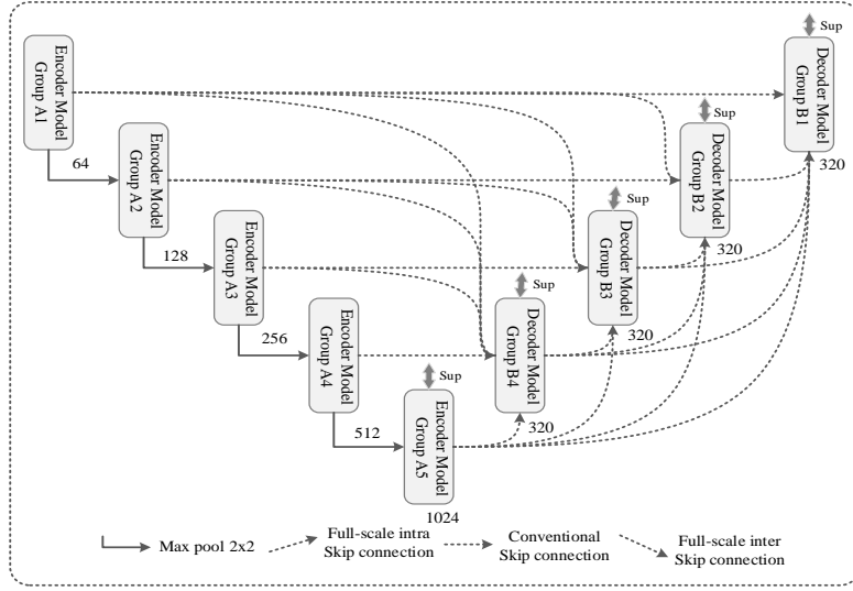
图 4. MSFCA-Unet 分割网络结构
