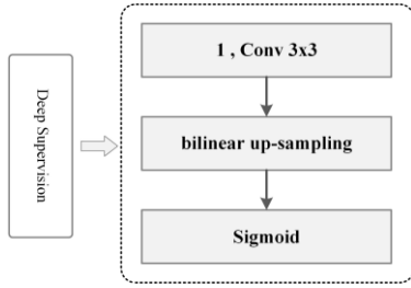
图 8. 深度监督模块结构
