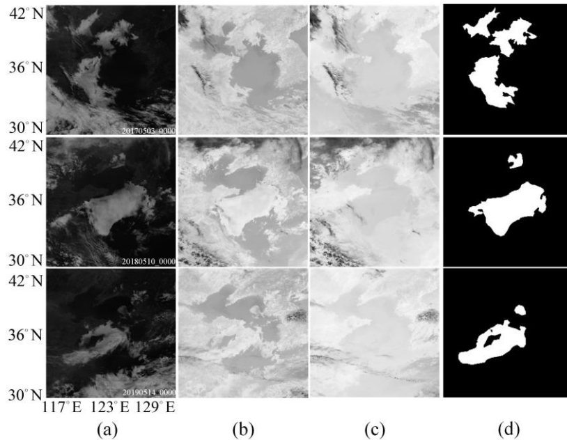
图 2. 所选取的云图通道及对应的海雾标签 (a) 通道 3(可见光波段, 0.64 \mu\text{m} ) (b) 通道 7(中红外波段, 3.9 \mu\text{m} ) (c) 通道 14(远红外波段, 11.2 \mu\text{m} ) (d) 海雾标签图
