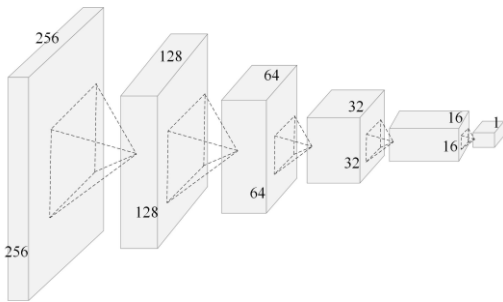
图 9. 判别器结构图
