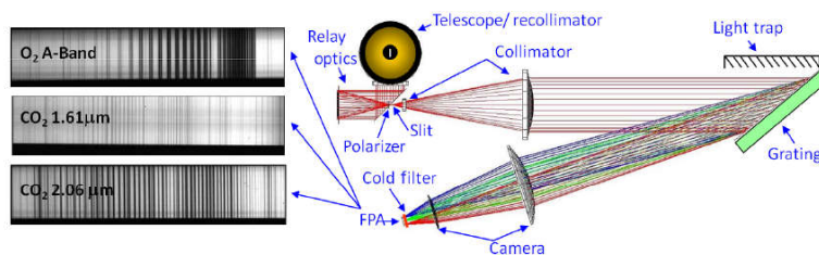
图 2 OCO 光学系统结构图
