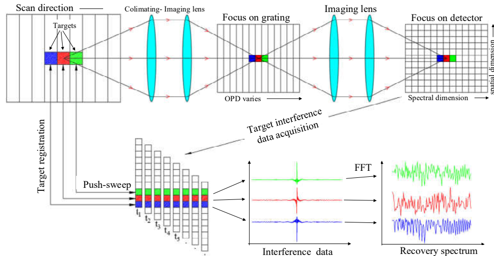
图 7 时空联合调制成像光谱仪信息获取过程示意图
