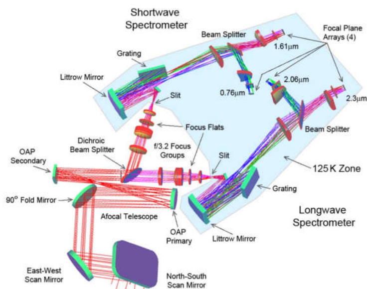
图 4 GeoCarb 光学系统结构图
