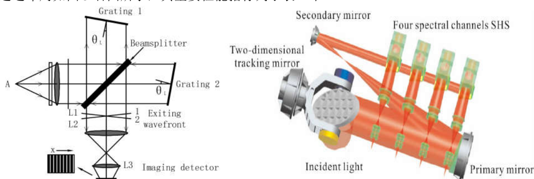
图 3 GMI 光学系统结构图
