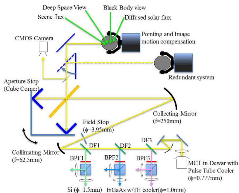
图 1 TANSO-FTS 光学系统结构图
