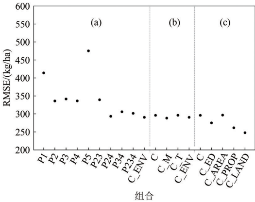
图5 不同组合随机森林验证结果 Fig. 5 Validation results of random forest with different combinations
