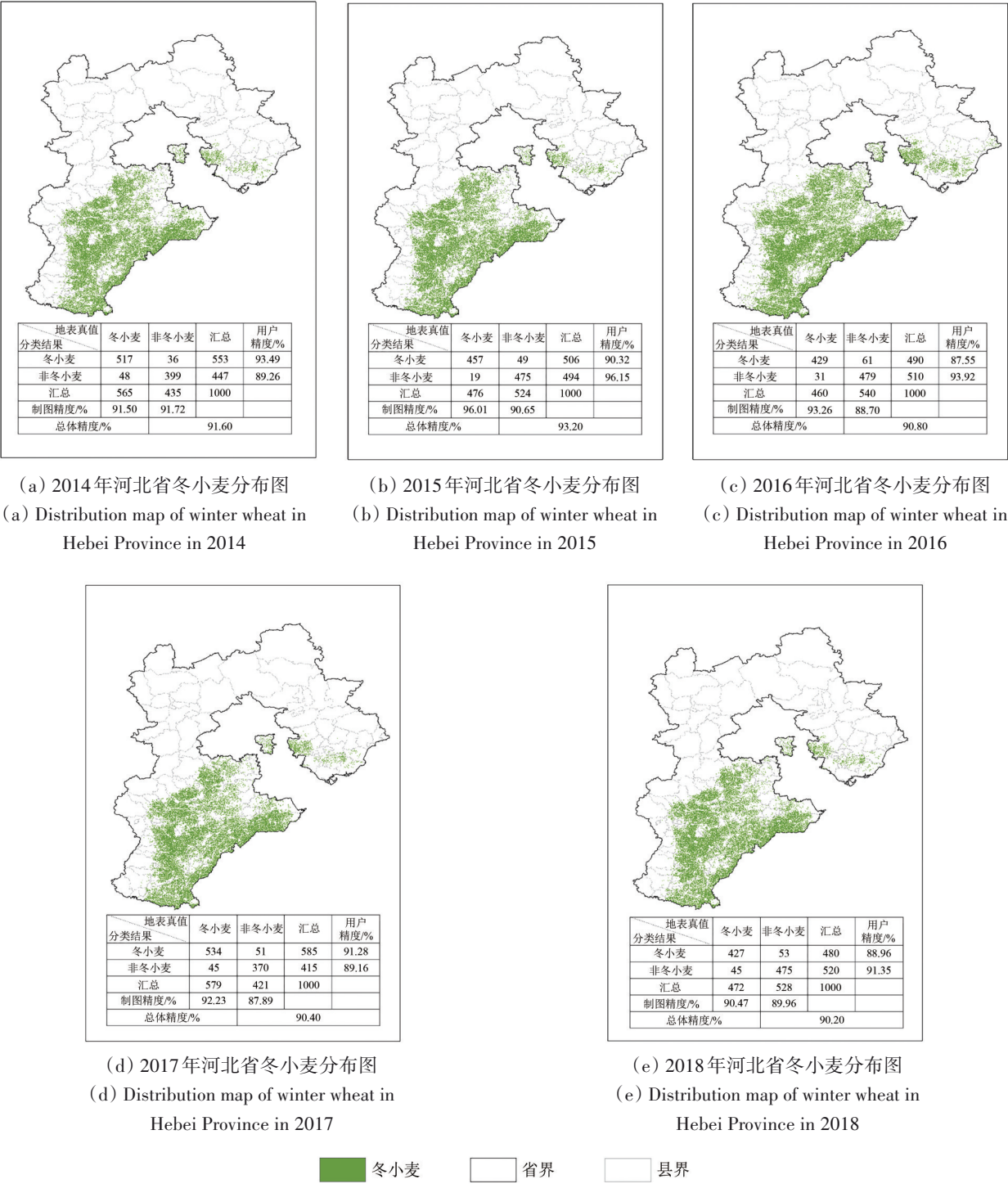
图2 河北省冬小麦种植分布图 Fig. 2 Distribution map of wheat in Hebei Province
